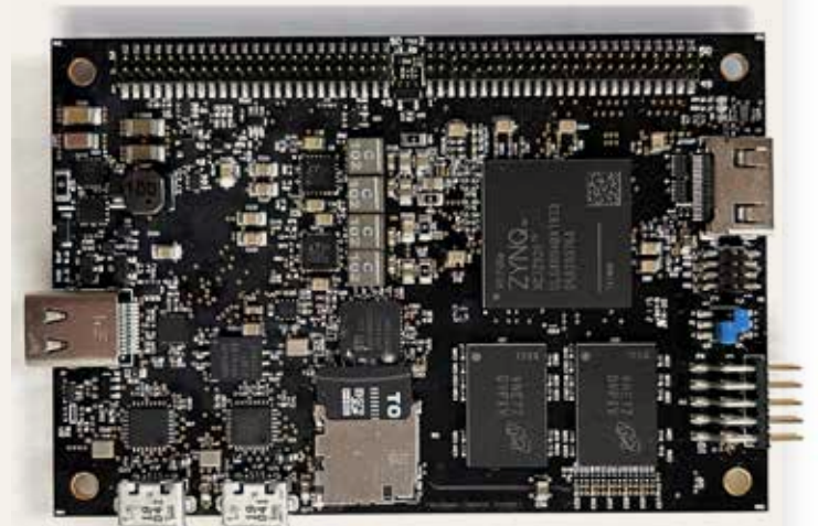
IoTプロセッサ-MSX3ボード
