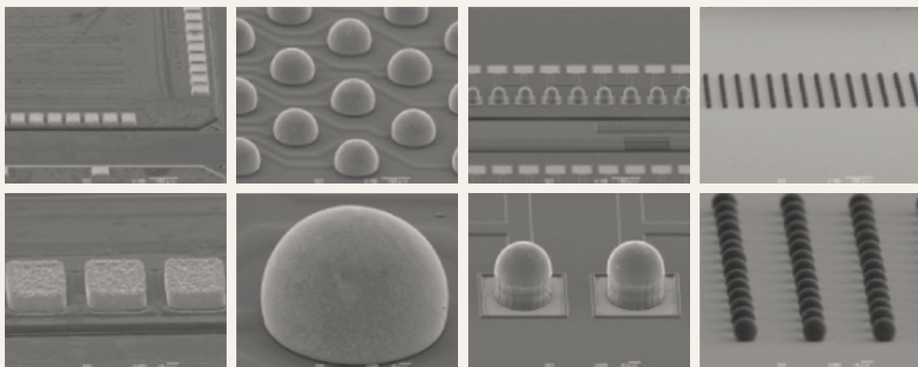
めっきで作製した金やはんだの電子回路実装用パンプ(微小な突起状の端子)
